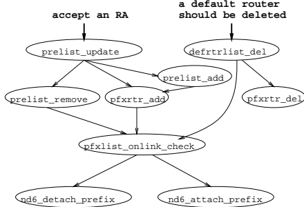
図 9 カーネル内での制御の流れ Fig. 9 Control flow in kernel
