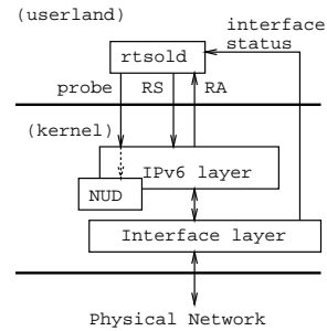
図 10 システム全体の構成 Fig. 10 System configuration
